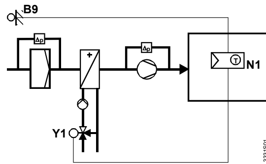
Raumtemperaturregelung durch Steuern des Heizventils, mit Aussentemperaturkompensation
